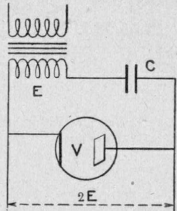
FIG. 6. - REDRESSEUR DOUBLANT LA TENSION
