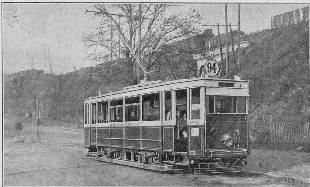
VOITURE DE TRAMWAY TYPE « To » AMÉNAGÉE POUR LE SERVICE A UN OU DEUX AGENTS
