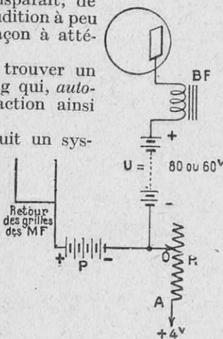
FIG. 1. - SCHEMA DU DISPOSITIF CORRECTEUR DE FADING
