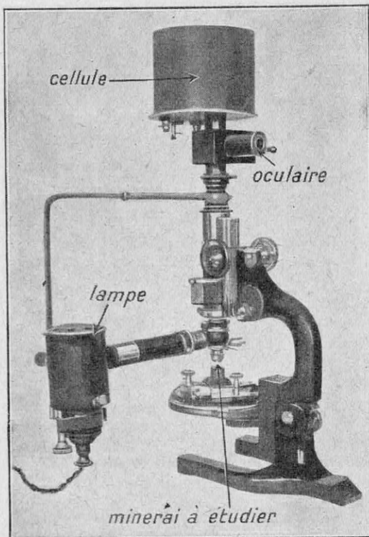
FIG. 9. — LE MICROSCOPE PÉTROGRAPHIQUE DE M. ORCEL, POUR L'ÉTUDE DES MINÉRAIS
