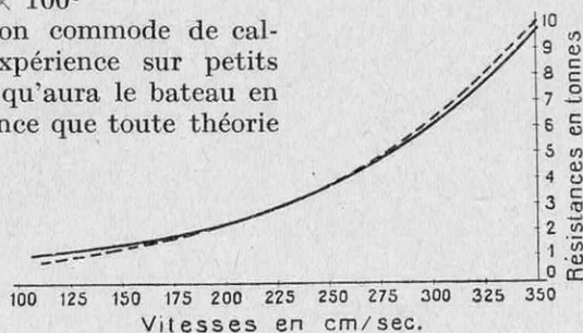
FIG. 3. — CES COURBES MONTRENT LA PRÉCISION QUE PEUT DONNER L'ÉTUDE D'UNE MAQUETTE DE CARÈNE
