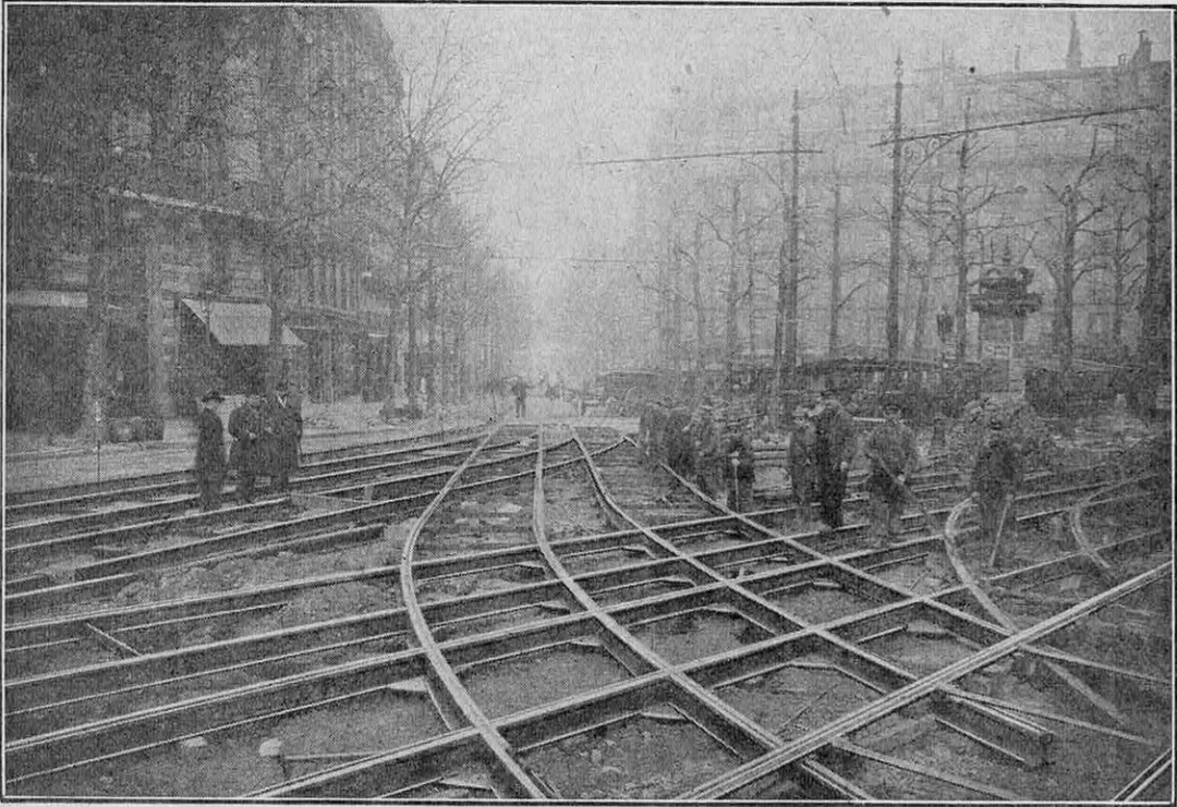
TRAVAUX DE VOIE AU CARREFOUR MICHEL-ANGE-AUTEUIL Mise en place d'un croisement entièrement construit en atelier.
