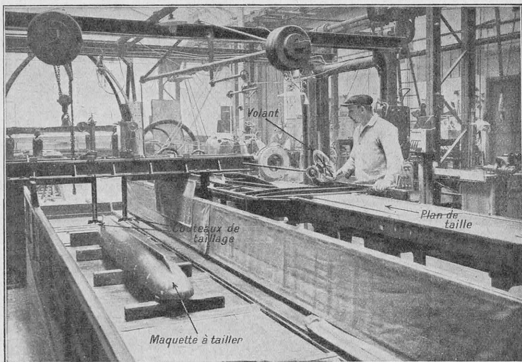
FIG. 2. — COMMENT ON TAILLE UNE MAQUETTE DE PARAFFINE AU « BASSIN DES CARÈNES » DE LA PORTE DE VERSAILLES, A PARIS
