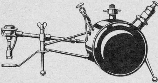
LE BRULEUR DE LABORATOIRES « PLUTON »
