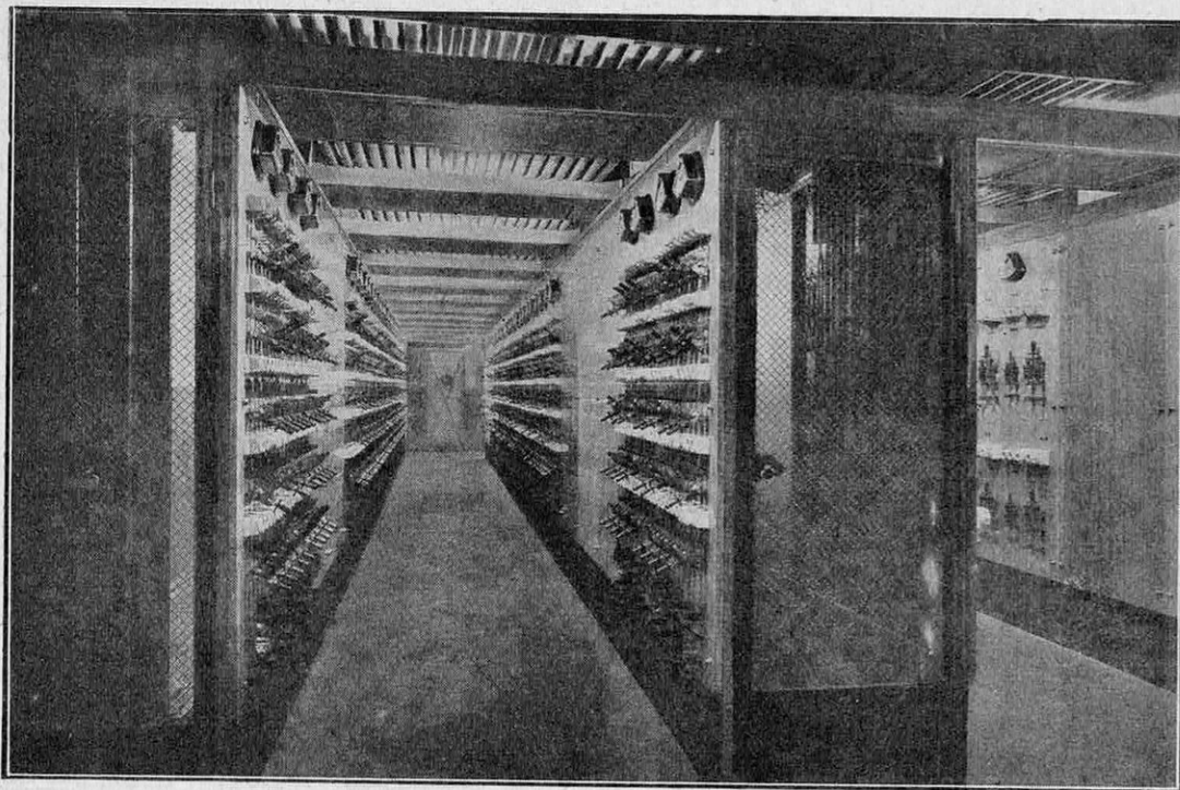
FIG. 6. — UN TABLEAU DE DISTRIBUTION COMPORTANT PRÈS DE 800 INTERRUPTEURS EST ALIMENTÉ PAR LE TABLEAU DE LA FIGURE 5 ET ASSURE L'ALLUMAGE, SUR DEMANDE TÉLÉPHONIQUE, DES RAYONS DES MAGASINS DE VENTE
