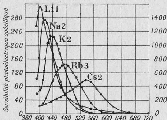
FIG. 4. — COURBES MONTRANT LA VARIATION DU COURANT PHOTOÉLECTRIQUE EN FONCTION DE LA LONGUEUR D'ONDE DE LA LUMIÈRE INCIDENTE
