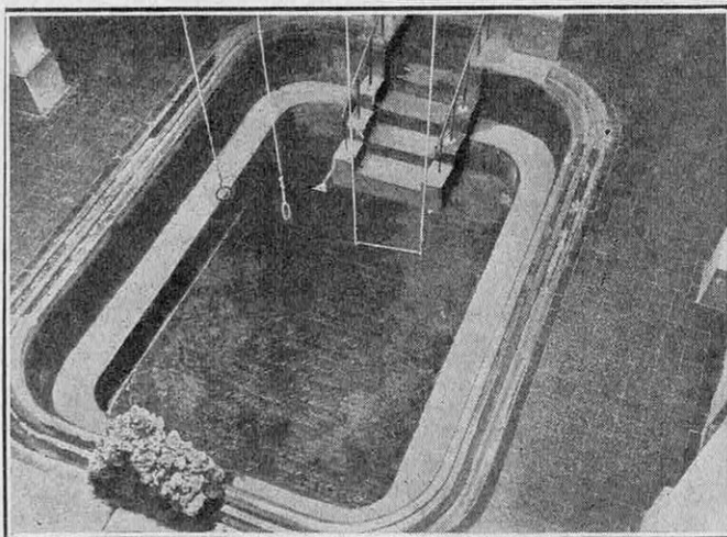
PISCINE GALLO-ROMAINE A AMÉLIE-LES-BAINS (PYR.-OR.) A l'intérieur, on aperçoit la banquette sur laquelle s'asseyaient les baigneurs.
