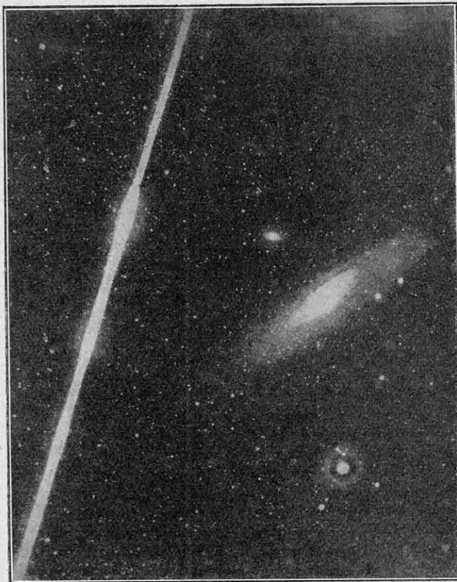
PHOTOGRAPHIE D'UN BOLIDE AU VOISINAGE DE LA NÉBULEUSE D'ANDROMÈDE
