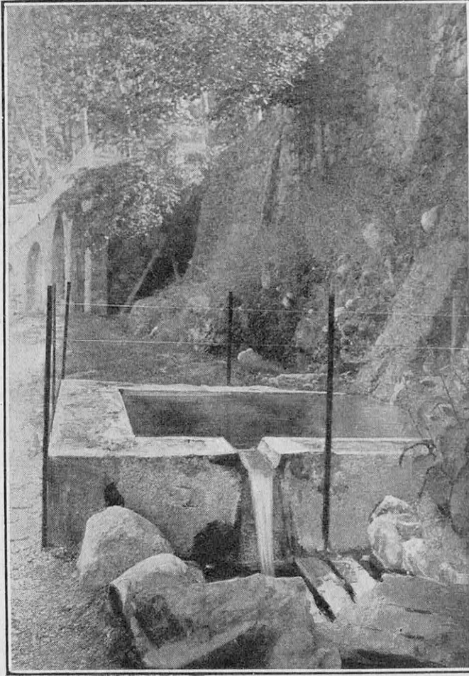
LA SOURCE CHAUDE SAINT-ANDRÉ, A THUEZ-LES-BAINS (PYRÉNÉES-ORIENTALES)
