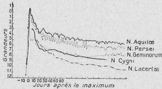
COURBES PHOTOMÉTRIQUES CARACTÉRISTIQUES DE DIVERSES NOVAE
