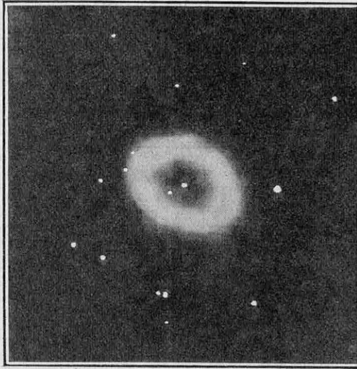
NÉBULEUSE ANNULAIRE DE LA LYRE, PHOTOGRAPHIÉE A L'OBSERVATOIRE DU MONT WILSON
