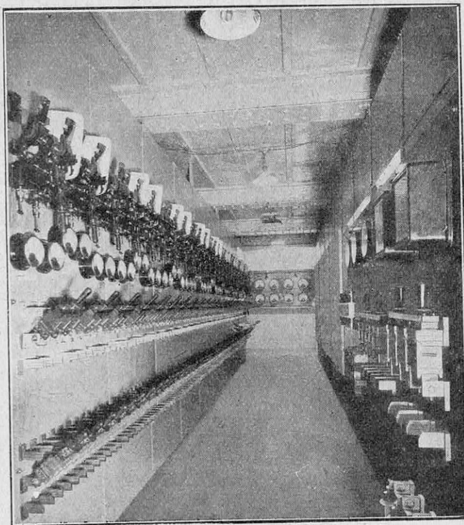
FIG. 5. — VUE DE L'UNE DES TROIS GALERIES DU TABLEAU DE DISTRIBUTION
