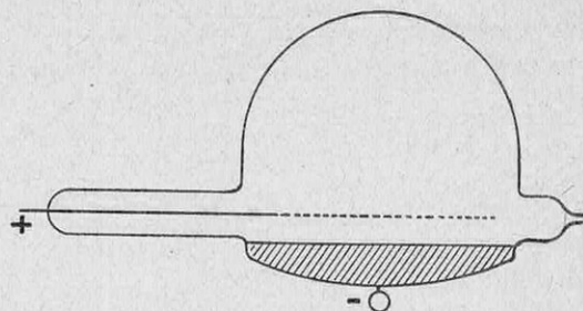
FIG. 2. — SCHÉMA D'UNE CELLULE PHOTOÉLECTRIQUE CONSTRUITE PAR LA GENERAL ELECTRIC COMPANY ANGLAISE
