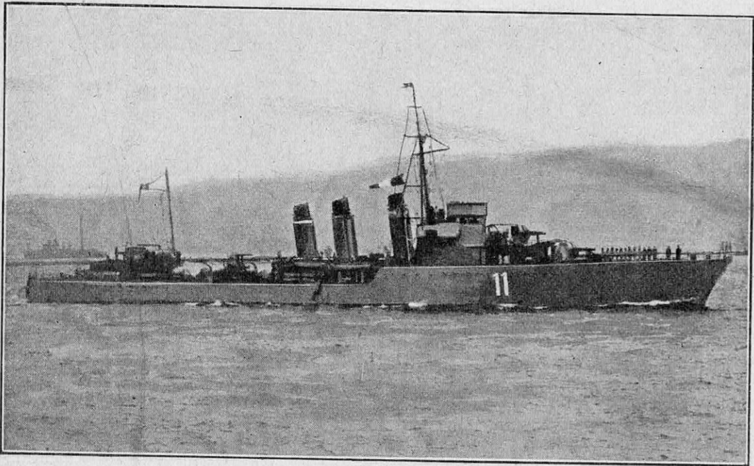
TORPILLEUR FRANÇAIS « TEMPÊTE » DE 1.340 TONNES ET 105 MÈTRES DE LONG, ARMÉ DE QUATRE PIÈCES DE 130, UNE DE 75 ANTIAÉRIENNE ET SIX TUBES LANCE-TORPILLES
