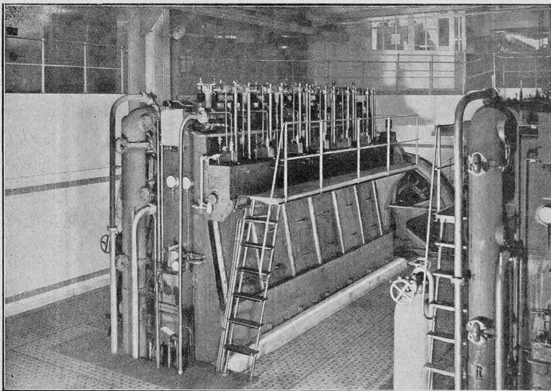
FIG. 3. — MOTEUR DIESEL A 6 CYLINDRES, A INJECTION MÉCANIQUE DU COMBUSTIBLE (MAZOUT OU HUILE DE GOUDRON) COMPRIMÉ A 250 KG PAR CENTIMÈTRE CARRÉ
