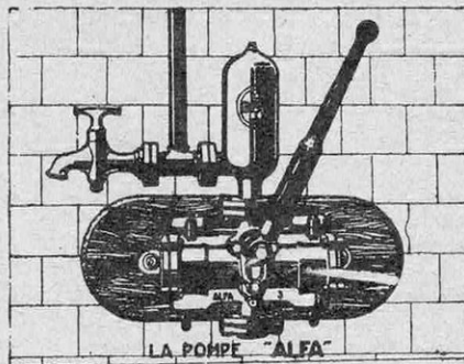
LA POMPE « ALFA », ASPIRANTE ET FOULANTE, A PISTON A DOUBLE EFFET ET A MOUVEMENT ALTERNATIF, EST D'UN FONCTIONNEMENT TRÈS DOUX
