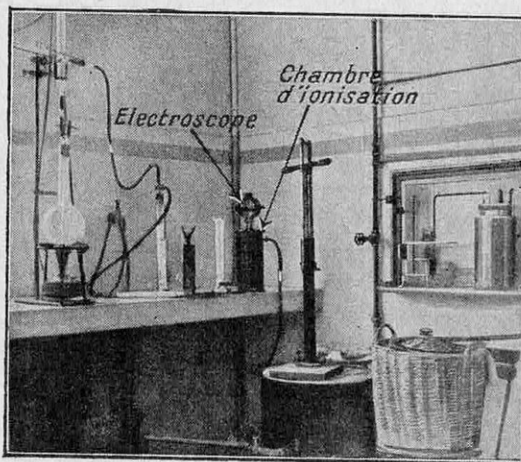
MESURE DE LA RADIOACTIVITÉ DES GAZ DE SOURCE THERMALE AU LABORATOIRE D'HYDROLOGIE (M. LÉPAPE)
