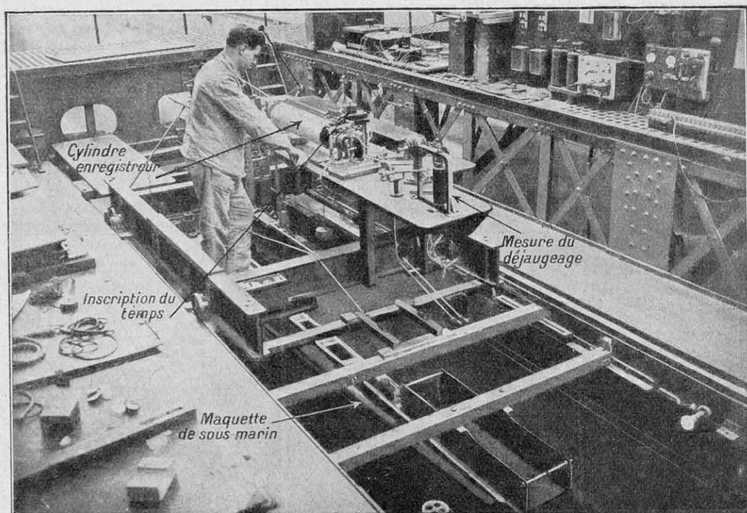
FIG. 6. — ÉTUDE D'UNE MAQUETTE DE SOUS-MARIN AU « BASSIN DES CARÈNES » DE PARIS Le pont roulant supporte tous les appareils enregistreurs nécessaires à l'étude des propriétés des maquettes. Il est également muni de l'appareillage indispensable à l'étude des hélices.
