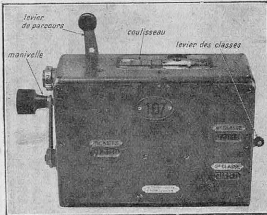
APPAREIL OBLITÉRATEUR-ENREGISTREUR ACCROCHÉ AU CEINTURON DU RECEVEUR
