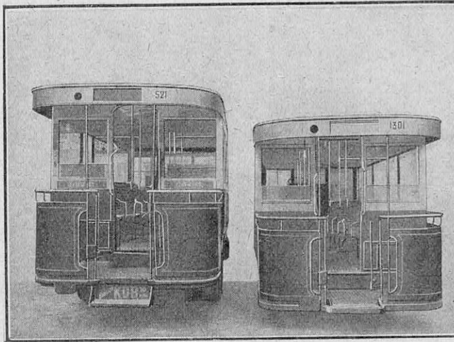
VUE ARRIÈRE DE DEUX AUTOBUS, L'UN A CHASSIS ORDINAIRE, L'AUTRE A CHASSIS SURBAISSÉ
