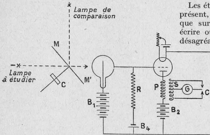
FIG. 7. — SCHEMA DE MONTAGE POUR LA COMPARAISON DE DEUX LAMPES, A L'ELECTRICAL TESTING LABORATORY, DE NEW YORK
