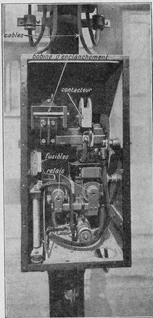
CONTACTEUR D'INTERCONNEXION MONTÉ SUR POTEAU
