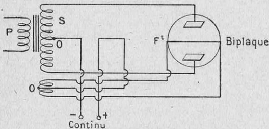
FIG. 5. - MONTAGE ORDINAIRE D'UN REDRESSEUR DE COURANT AVEC VALVE BIPLAQUE
