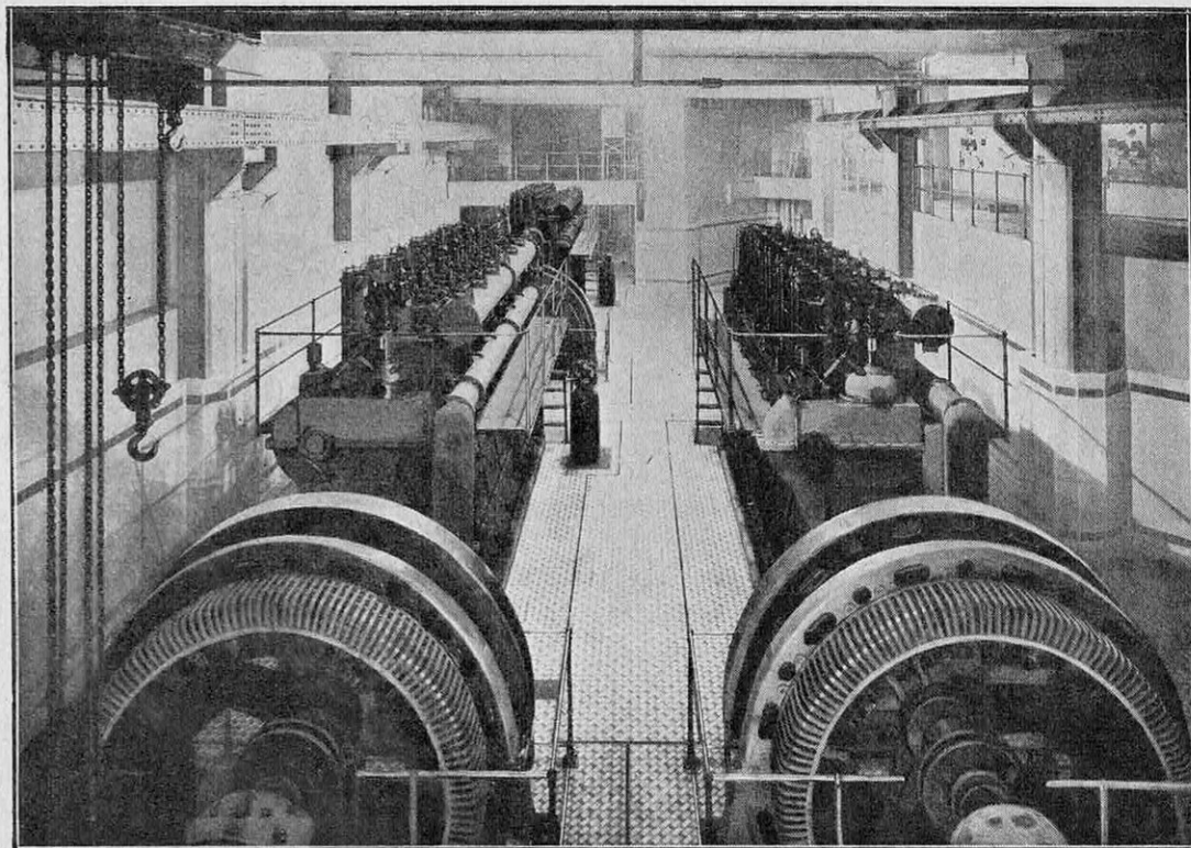
FIG. 2. — ENSEMBLE DE LA SALLE DES MACHINES AVEC LES TROIS GROUPES ÉLECTROGÈNES A MOTEURS DIESEL DE 650 CH CHACUN, VU DU PUPITRE DE COMMANDE REPRÉSENTÉ FIG. 4.
