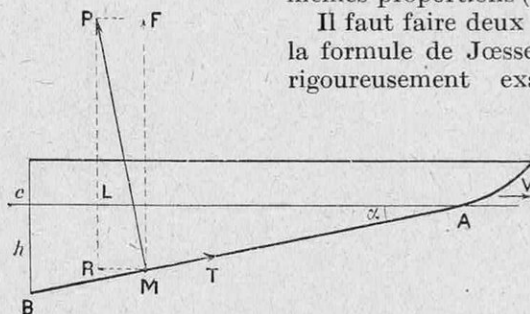
FIG. 5. — DONNER AUX NAVIRES LA FORME D'UN GLISSEUR PERMETTRAIT D'ATTEINDRE ÉCONOMIQUEMENT DE GRANDES VITESSES
