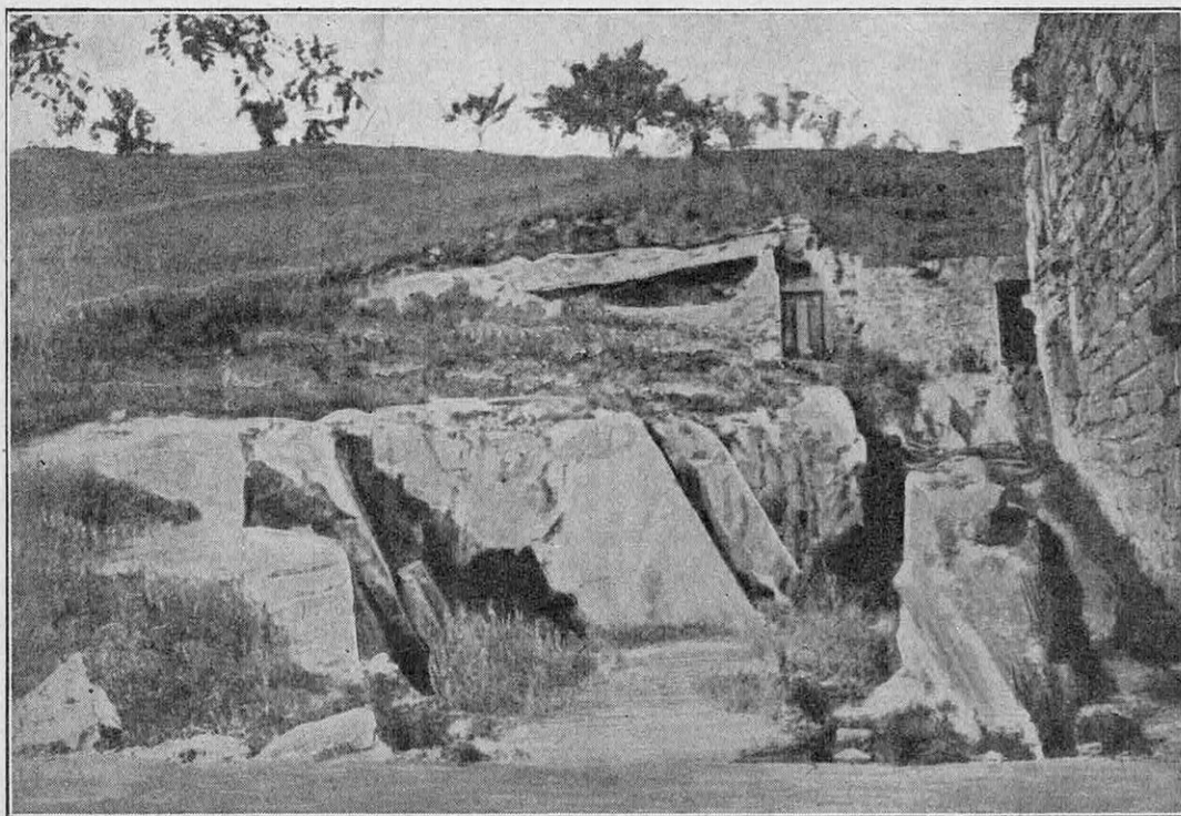
EMERGENCE DES FAILLES GRANITIQUES A L'ENTRÉE DES GALERIES DES SOURCES PAPON, A SAINT-NECTAIRE (PUY-DE-DÔME)
