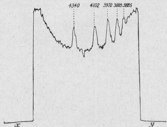
FIG. 8. — COURBE SPECTRALE DE L'ÉTOILE VÉGA, OBTENUE AVEC LE MICROPHOTOMÈTRE ENREGISTREUR CHALONGE ET LAMBERT
