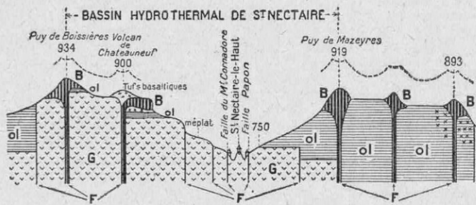
COUPE VERTICALE DE LA CHAINE DES DOMES, AUX ABORDS DE SAINT-NECTAIRE (PUY-DE-DÔME)
