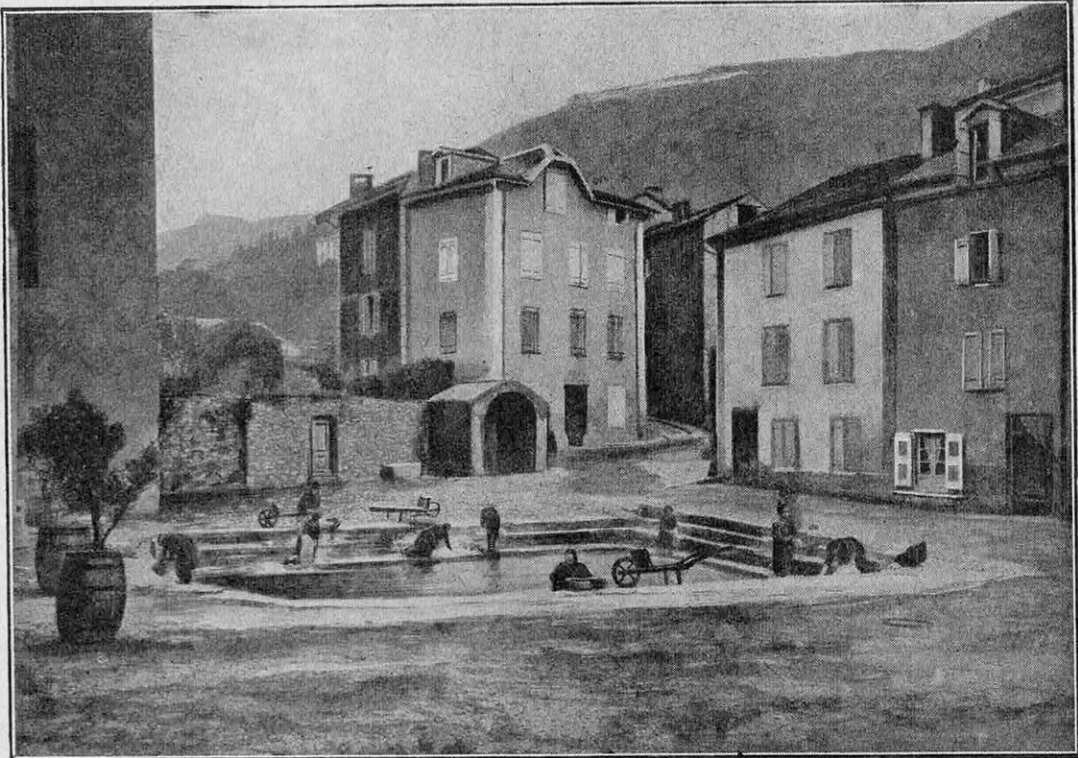
SOURCE THERMALE SUR UNE PLACE PUBLIQUE A AX-LES-THERMES (ARIÈGE) THERMAL SPRING ON A PLACE AT AX-LES-THERMES (ARIÈGE)
