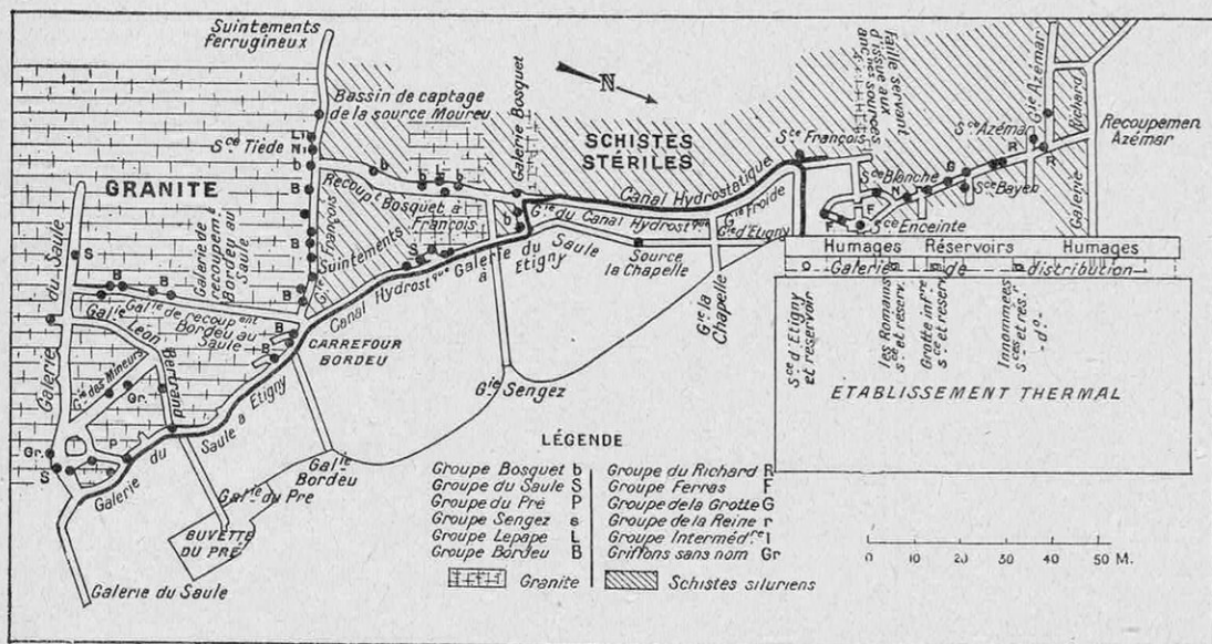
COUPE HORIZONTALE DE LA MONTAGNE AUX ABORDS DE L'ÉTABLISSEMENT THERMAL DE BAGNÈRES-DE-LUCHON (HAUTE-GARONNE)
