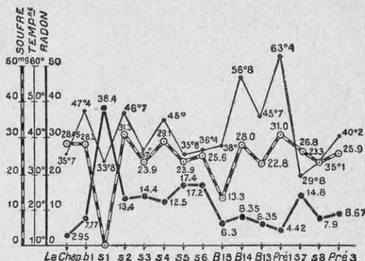
GRAPHIQUE OBTENU PAR M. LEPAPE, MONTRANT LA RELATION DE LA SULFURATION DES SOURCES AVEC LEUR RADIOACTIVITÉ
