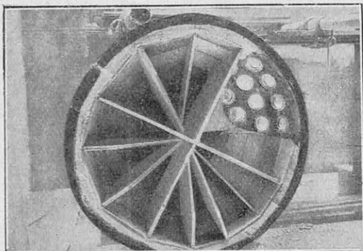
QUELQUES-UNES DES OPÉRATIONS NÉCESSAIRES POUR LA CONSTRUCTION D'UNE COUPOLE EN BÉTON TRANSLUCIDE, AVEC PAVÉS DE VERRE ROUNDS
