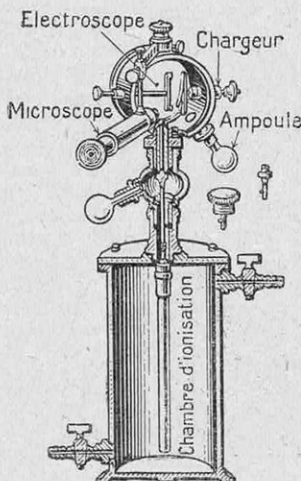
I. ÉLECTROSCOPE P. CURIE
