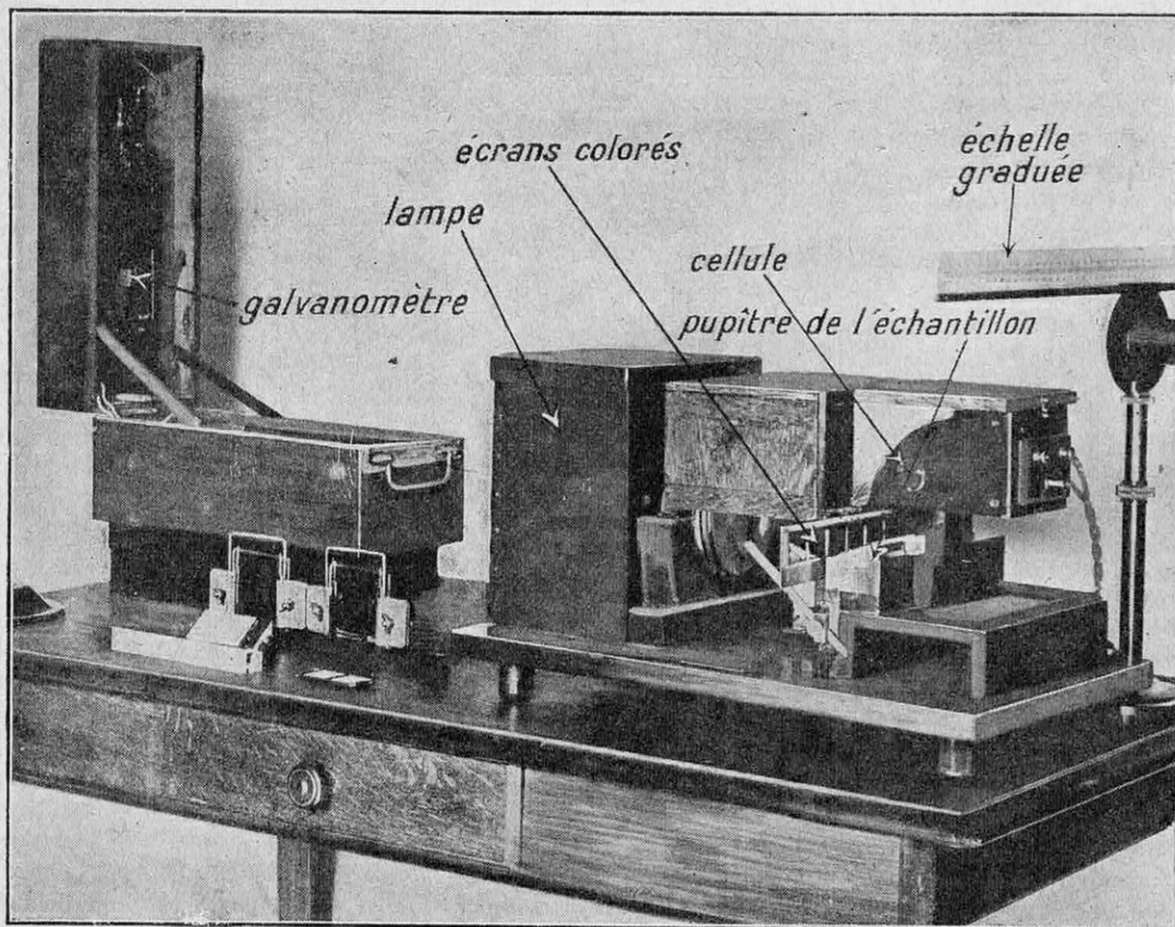
FIG. 10. — VUE DU COLORIMÈTRE T. C. B. A CELLULE PHOTOÉLECTRIQUE, QUI PERMET D'Étudier LA COULEUR D'UN Échantillon DE PAPIER OU D'Étoffe, OU DE COMPARER DEUX Échantillons ENTRE EUX
