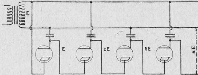
FIG. 9. — ON PEUT ÉLEVER LA TENSION AUTANT DE FOIS QU'ON LE DÉSIRE EN MULTIPLIANT LES ÉTAGES
