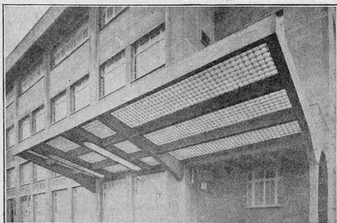
MARQUISE A L'AÉROPORT DU BOURGET, PRÈS PARIS, CONSTRUITE EN BÉTON TRANSLUCIDE
