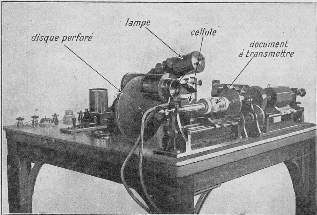
FIG. 14. — VUE D'ENSEMBLE D'UN POSTE TRANSMETTEUR ED. BELIN EMPLOYÉ POUR LA TÉLÉPHOTOGRAPHIE
