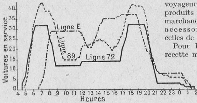
COMMENT VARIE LE NOMBRE DES VOITURES SUIVANT LES HEURES DE LA JOURNÉE
