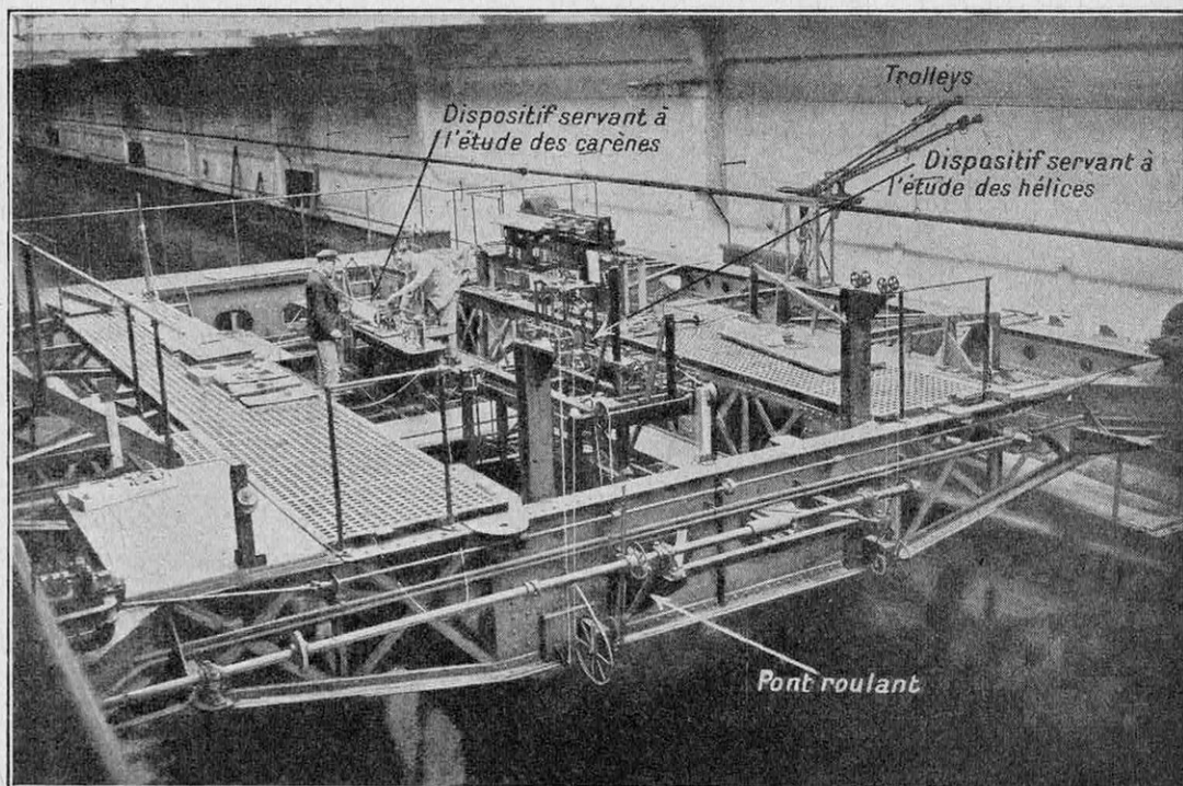
FIG. 4. — LE « BASSIN DES CARÈNES » DE PARIS ET LE PONT ROULANT AU-DESSOUS DUQUEL EST FIXÉE LA MAQUETTE DU NAVIRE A ÉTUDIER
