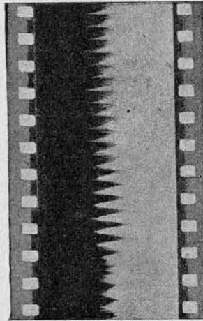
FIG. 12. — FILM SONORE ENREGISTRÉ PAR LE PROCÉDÉ A DENSITÉ CONSTANTE
