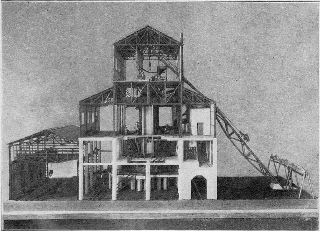
TYPE D'UNE INSTALLATION DE HAUT FOURNEAU ÉLECTRIQUE DESSERVIE PAR UNE USINE HYDRAULIQUE, EN SUÈDE
