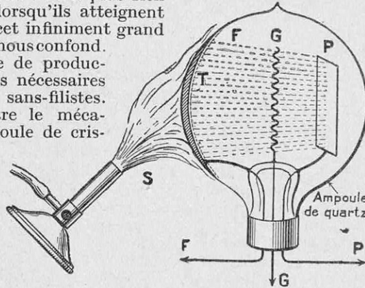
FIG. 3. — SOLUTION THERMIQUE DE LA LAMPE SANS FILAMENT
