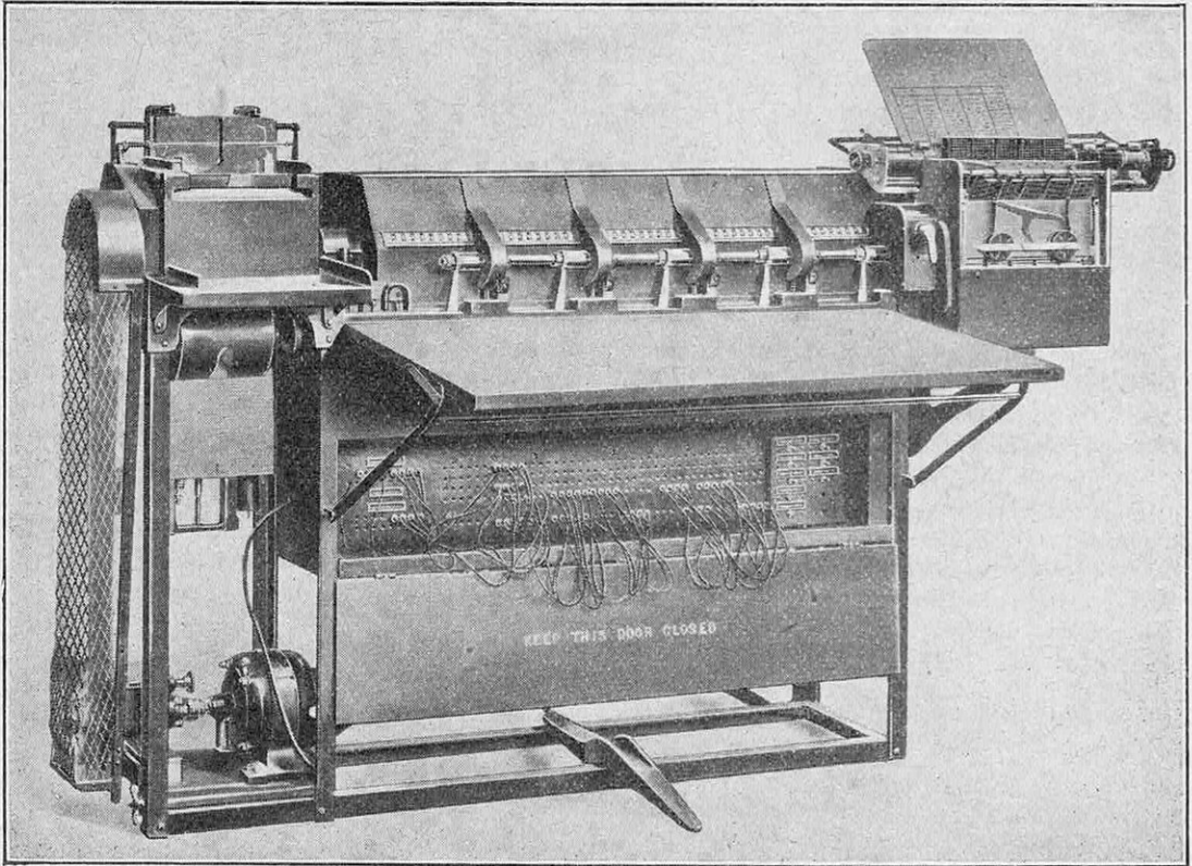
MACHINE ÉLECTRIQUE QUI ANALYSE LES INDICATIONS PORTÉES SUR LES CARTES
