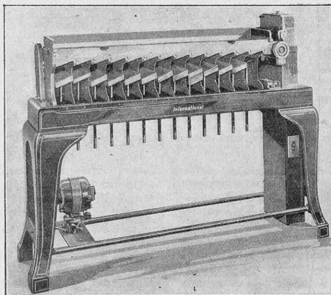
TRIEUSE ÉLECTRIQUE POUR LE CLASSEMENT DES CARTES
