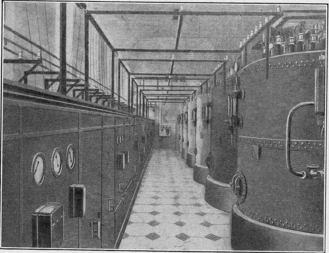
LA PLUS PUISSANTE INSTALLATION DE CHAUDIÈRES ÉLECTRIQUES DU MONDE Cette installation, aux papeteries de Wargon, absorbe 25.000 chevaux et fonctionne en parallèle avec un accumulateur de vapeur Rutles.
