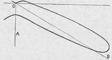
FIG. 10 ET 11. — POUR QUE L'ÉCLAIRAGE SOIT LE MÊME EN « A » ET « B », IL FAUT QUE L'INTENSITÉ LUMINEUSE SOIT HUIT FOIS PLUS FORTE DANS LA DIRECTION « O B » QUE DANS LA DIRECTION « O A »
