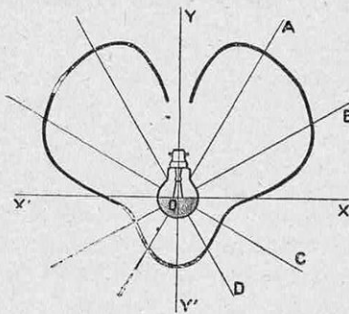
FIG. 9. — UNE LAMPE SEMI-ÉMAILÉE OU DÉPOLIE DU CÔTÉ OPPOSÉ AU CULOT, RÉALISE UN ÉCLAIRAGE SEMI-INDIRECT C'est pourquoi on ne doit pas employer de telles lampes dans un espace découvert ou dans un espace couvert avec plafond sombre, sans la placer dans un réflecteur.
