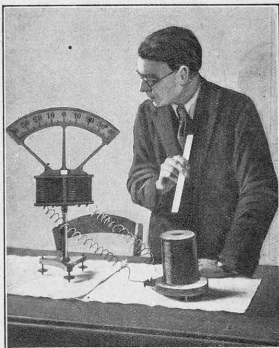
EXPÉRIENCE DE FARADAY SUR L'INDUCTION En approchant un aimant d'une bobine on produit un courant qui fait dévier un galvanomètre
