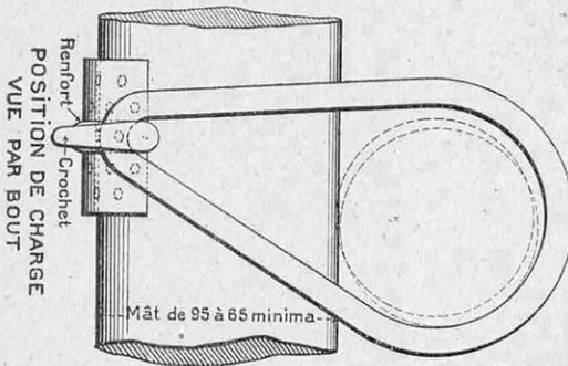
AGRAFE POUR MATS
