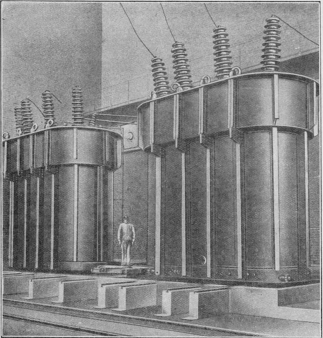
DEUX TRANSFORMATEURS DE 20.000 KILOWATTS CHACUN, A L'USINE DE VÅSTERAS
