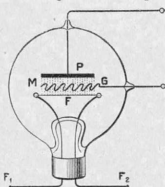
FIG. 1. — L'ÉMISSION ÉLECTRONIQUE D'UNE VALVE A TROIS ÉLECTRODES
