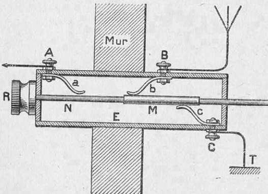
FIG. 8. — DISPOSITIF DE MISE A LA TERRE
