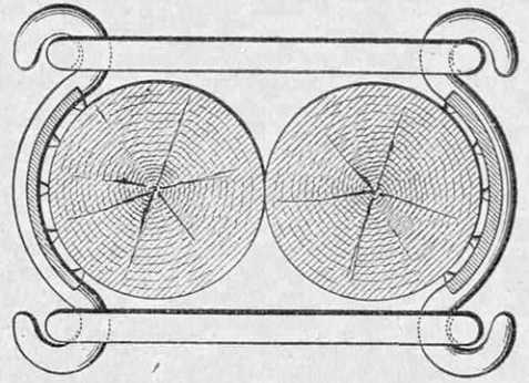
JUMELAGE DE DEUX MATS VERTICAUX PAR NŒUD INSTANTANÉ
