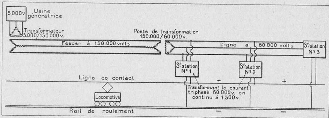
SCHÉMA D'INSTALLATION ÉLECTRIQUE DES CHEMINS DE FER FRANÇAIS
