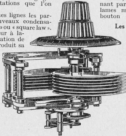
ENSEMBLE DU CONDENSATEUR BARDON, SUIVANT LA « LOI DU CARRÉ »
