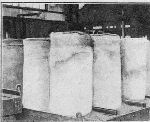
FIG. 3. — CYLINDRES DE CYANAMIDE A LA SORTIE DU FOUR D'AZOTURATION
