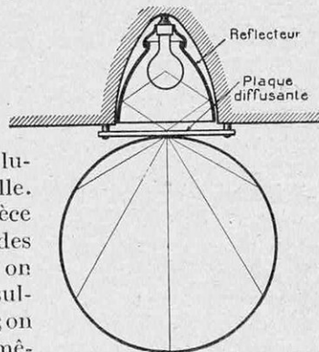
FIG. 5. — ÉCLAIRAGE DIRECT AVEC RÉFLECTEUR ENCASTRÉ DANS LE PLAFOND ET PLAQUE DIFFUSANTE
