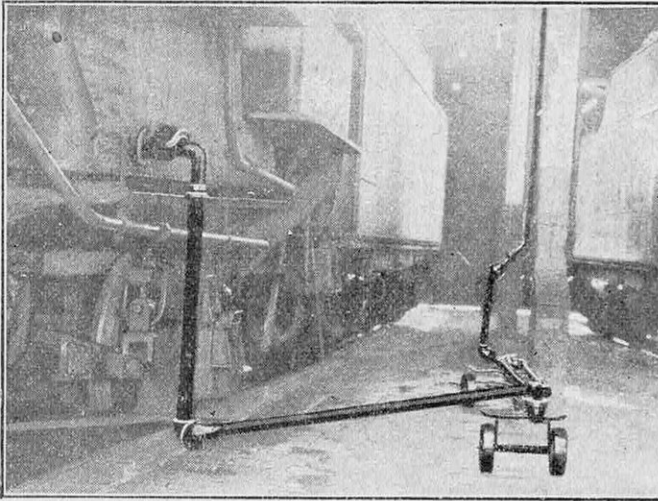
UN NOUVEAU DISPOSITIF POUR NETTOYER LES CHAUDIÈRES DE LOCOMOTIVES
