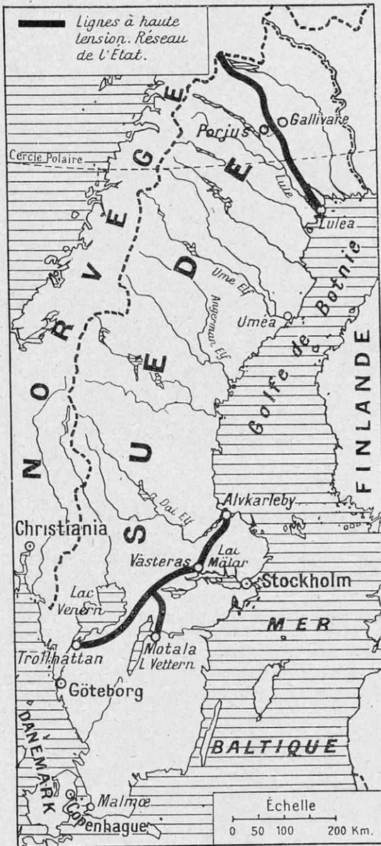
CARTE MONTRANT LA SITUATION DES LIGNES A HAUTE TENSION DE L'ÉTAT SUÉDOIS
