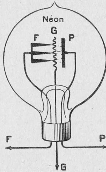
FIG. 5. — SOLUTION DE LA LAMPE SANS FILAMENT PROPOSÉE PAR L'AUTEUR
