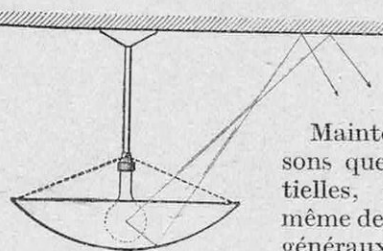
FIG. 7. — ÉCLAIRAGE INDIRECT PAR COUPE OPAQUE
