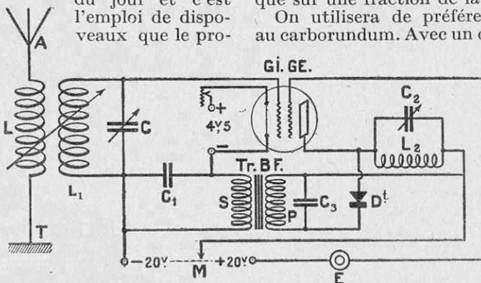
FIG. 6. — MONTAGE RÉFLEXE A LAMPE BIGRILLE A DÉTECTION PAR CRISTAL
