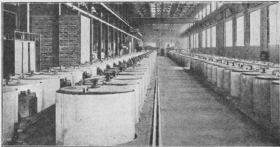
FIG. 2. — FOURS CYLINDRIQUES D'AZOTURATION DU CARBURE DE CALCIUM POUR OBTENIR LA CYANAMIDE
