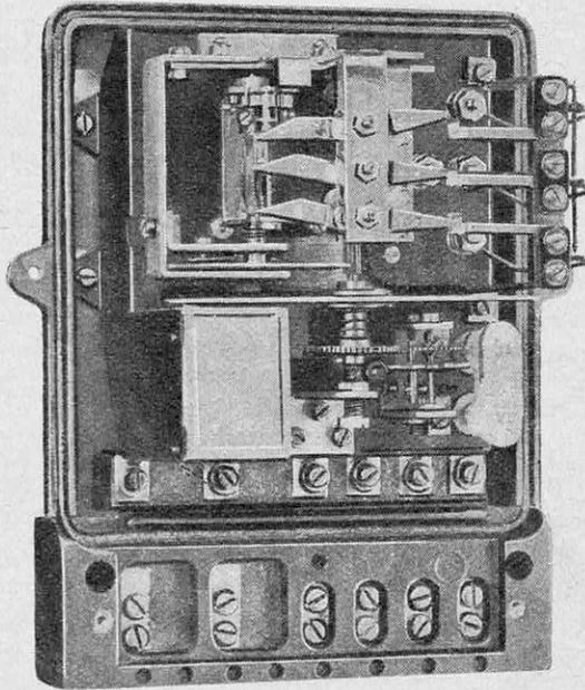
LE RELAIS A TRIPLE TARIF
