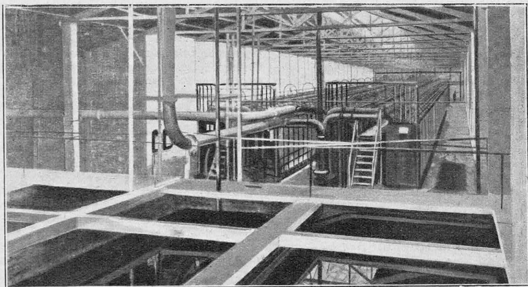
FIG. 4. — BATTERIE D'ÉLECTROLYSEURS SERVANT A PRÉPARER L'HYDROGÈNE UTILISÉ POUR LA SYNTHÈSE DE L'AMMONIAQUE
