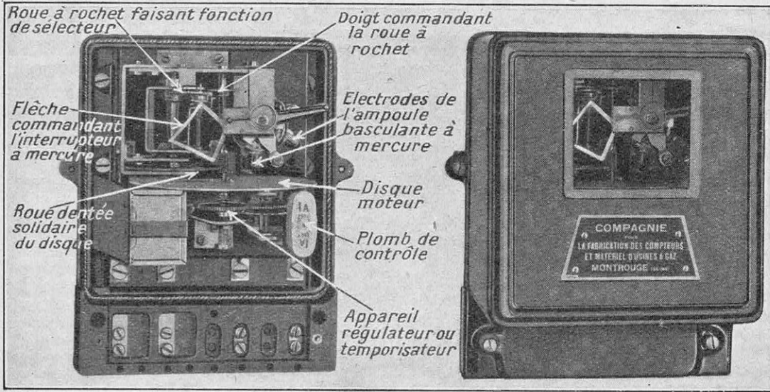
LE RELAIS SÉLECTEUR DE MANŒUVRE. APPAREIL OUVERT ET FERMÉ
