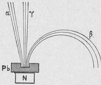
FIG. 2. — ÉMISSION D'UNE MATIÈRE RADIOACTIVE ANALYSÉE PAR UN CHAMP MAGNÉTIQUE
