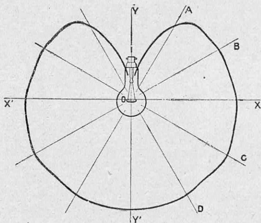
FIG. 2. - COURBE PHOTOMÉTRIQUE D'UNE LAMPE A ATMOSPHÈRE GAZEUSE A FILAMENT EN C
