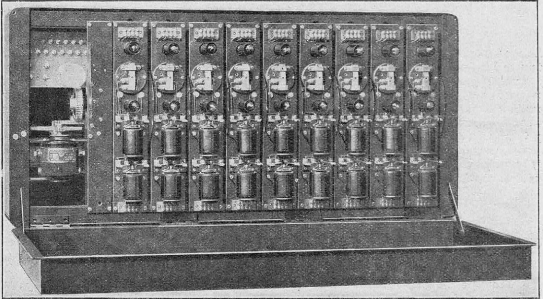
L'ÉMETTEUR AUTOMATIQUE DE SIGNAUX OUVERT
