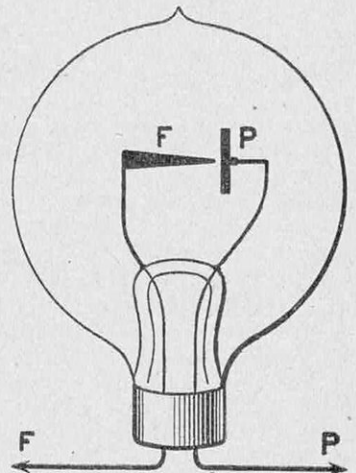
FIG. 4. — SOLUTION ÉLECTROSTATIQUE DU KÉNOTRON SANS FILAMENT
